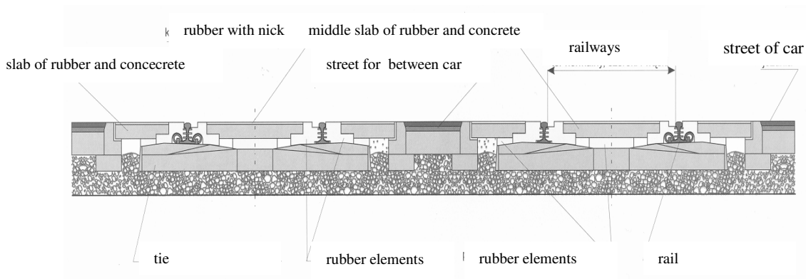
Fig. 4. Technical conception of vibroisolated railway crossing Rys. 4. Koncepcja techniczna wibroizolowanego przejazdu kolejowego
