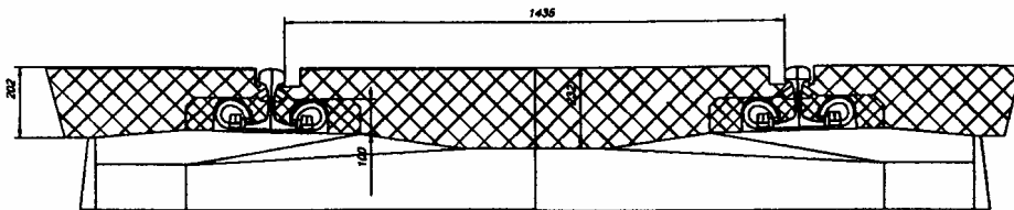
Fig. 7. Formed elastomer plate Rys. 7. Formowana płyta wykonana z elastomeru
