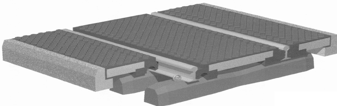
Fig. 8. Prototype of vibroisolated railroad crossing Rys. 8. Prototyp wibroizolowanego przejazdu kolejowego
