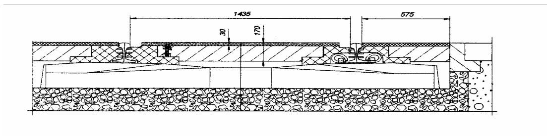
Fig. 5. Prefabricated concrete slab covered in elastomer anti-slide layer Rys. 5. Prefabrykowana płyta betonowa pokryta przeciwpoślizgową warstwą elastomerową
