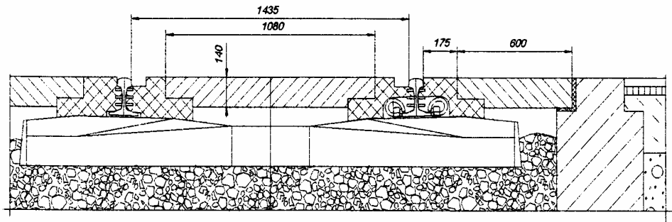
Fig. 6. Prefabricated concrete slab without elastomer anti-slide layer Rys. 6. Prefabrykowana płyta betonowa bez warstwy przeciwpślizgowej
