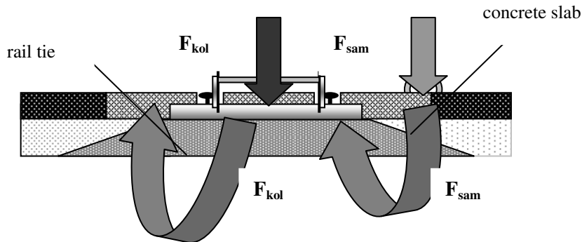
Fig. 1. Demonstration scheme of the influence of railroad and automotive vehicles on a traditional crossing Rys. 1. Rysunek poglądowy oddziaływania pojazdów szynowych i samochodowych na tradycyjny przejazd
