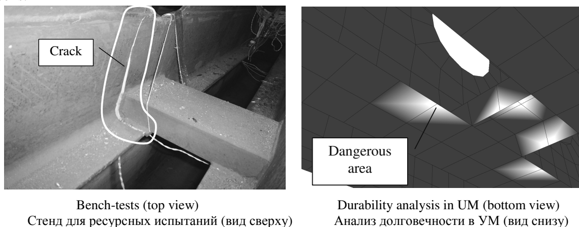
Fig. 5. Comparison: the crack from the bench test and the dangerous area from durability analysis Рис. 5. Сравнение: трещина в раме платформы после стендовых ресурсных испытаний и положение опасных точек после анализа долговечности
