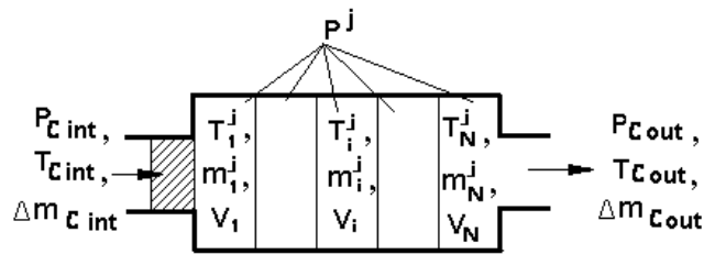
Fig. 5. The rated circuit design of volume of a cell to the beginning of the rated step Рис. 5. Схема рассматриваемого объема в начале номинального шага
