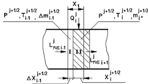
Fig. 6. The rated circuit design of i -th layer in the end of the first stage of a rated step Рис. 6. Схема для i -го слоя в конце первого этапа номинального шага
