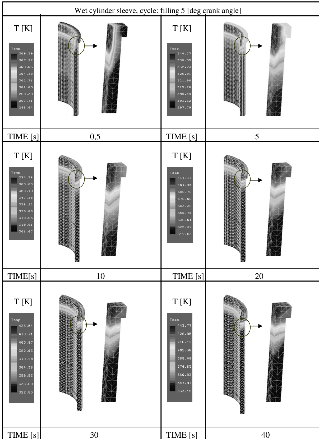
Fig. 2. Distribution of temperature in the wet cylinder sleeve Rys. 2. Rozkład temperatury w mokrej tulei cylindrowej
