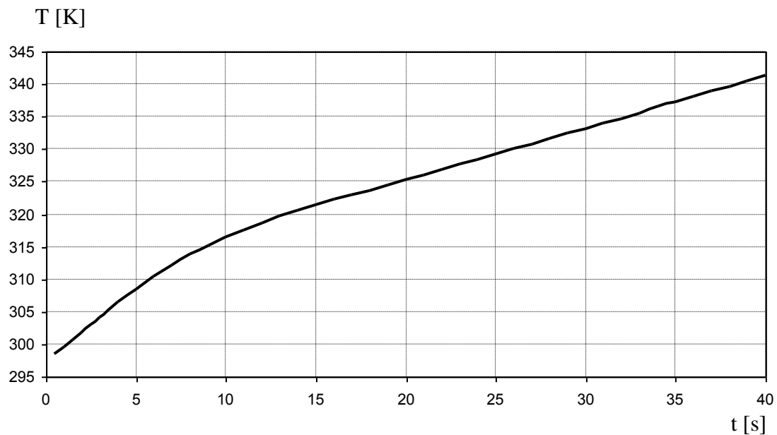
Fig. 5. The graph of changes average temperature on surface no. 3 Rys. 5. Wykres zmian średniej temperatury na powierzchni nr 3
