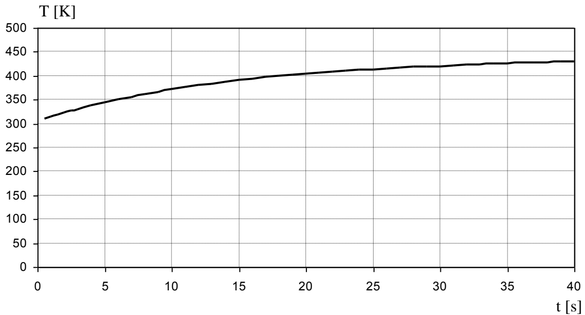
Fig. 3. The graph of changes average temperature on surface no. 1 Rys. 3. Wykres zmian średniej temperatury na powierzchni nr 1
