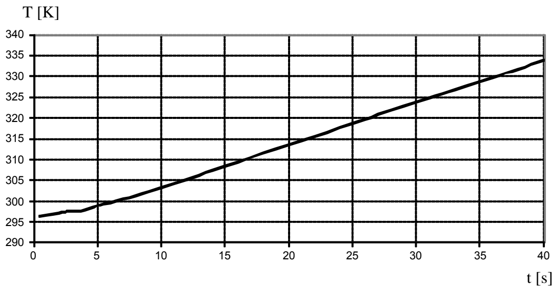
Fig. 6. The graph of changes average temperature on surface no. 4 Rys. 6. Wykres zmian średniej temperatury na powierzchni nr 4
