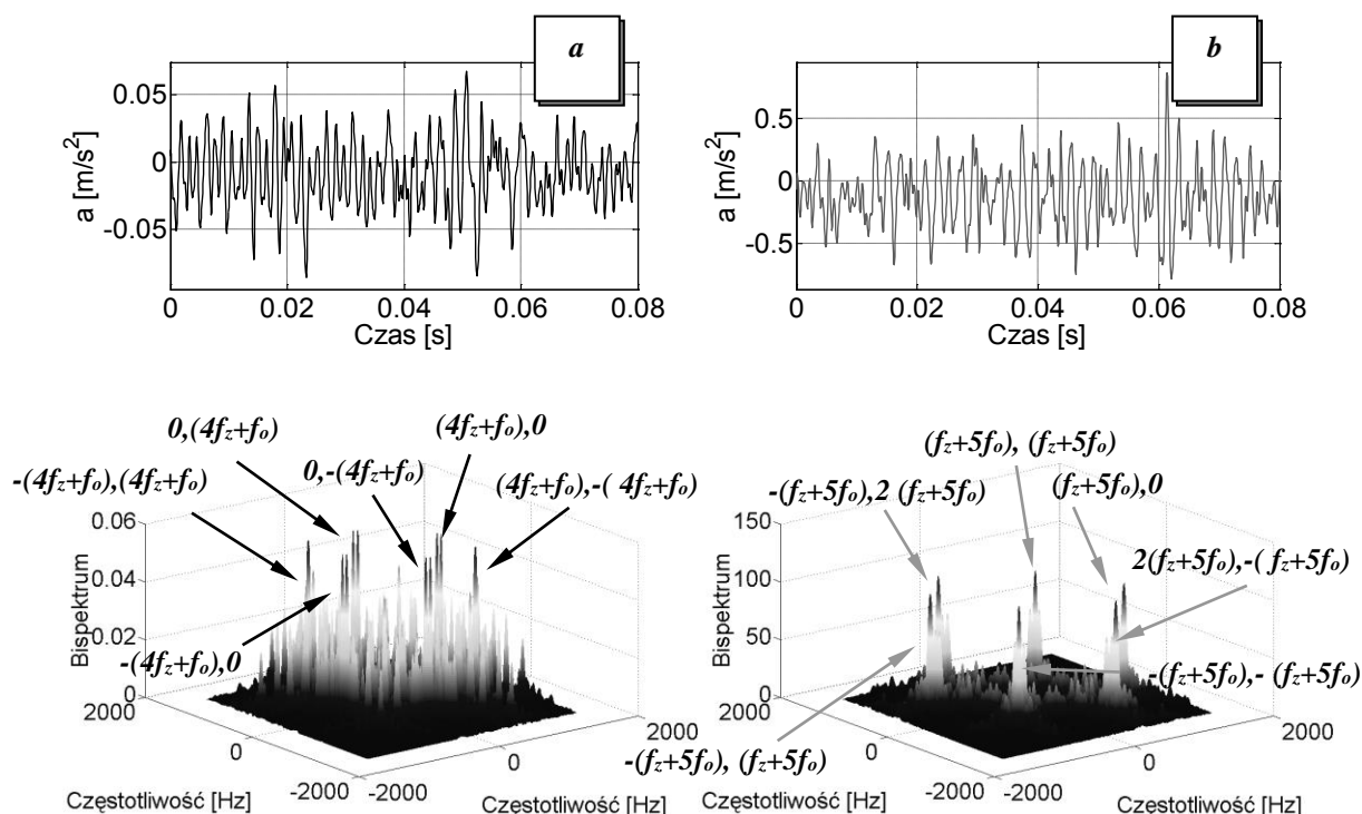
Rys. 4. Przebiegi czasowe oraz rozkłady bispektrum drgań przekładni zębatach napędów klatek walcowniczych w czasie pracy na luzie: a – przekładnia w ogólnym stanie dynamicznym dobrym (klatka k4), b – przekładnia przeznaczona do remontu (klatka k12)
