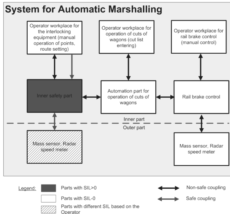
Fig. 5. Safety Distribution in the System for Automatic Split-up Activities Rys. 5. Rozkład bezpieczeństwa w systemie do czynności automatycznego rozdziału
