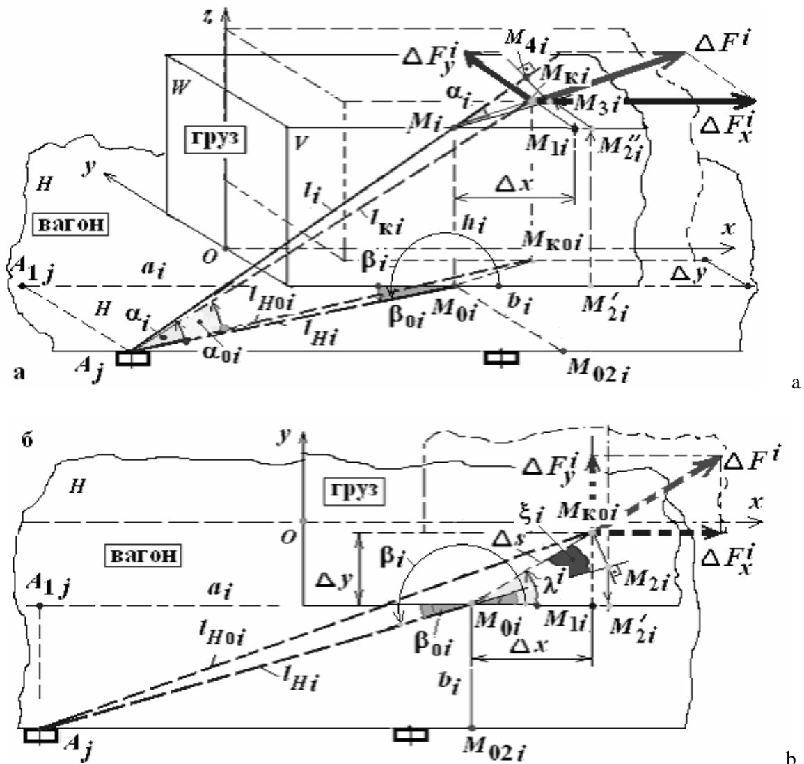
Fig. 2. General modelling cargoes displacement: a) – axonometric; b) – top view Рис. 2. Обобщённая модель сдвига груза: а) – аксонометрия; б) – вид сверху
