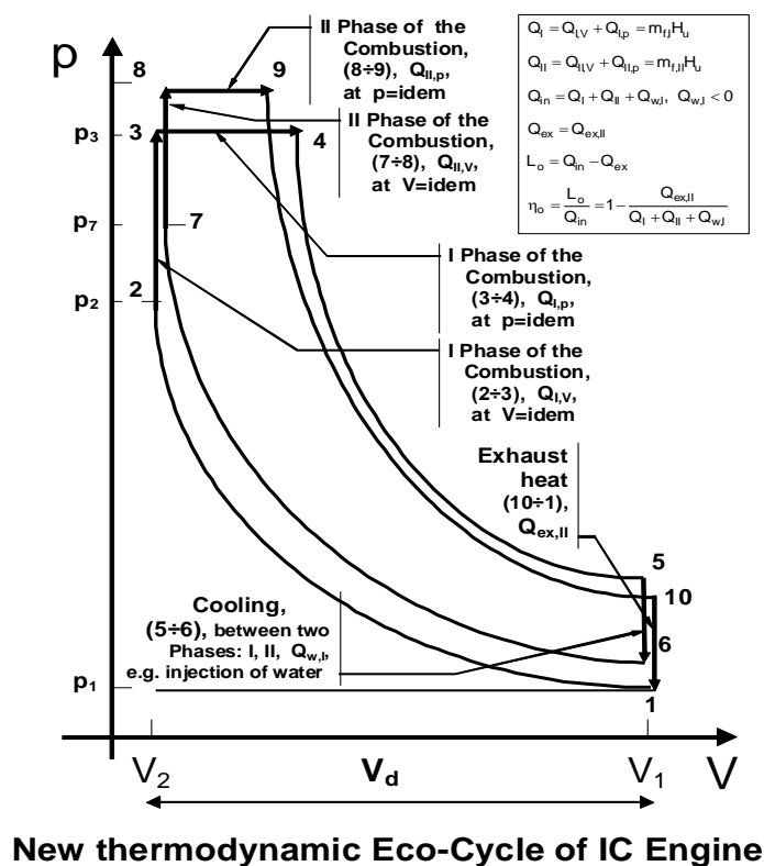
Fig. 10. Full composition of the thermodynamic reference eco-cycle Rys. 10. Pełny obraz termodynamicznego ekoobiegu porównawczego
