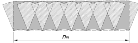
Fig. 2. Schematic diagram of minimum resolution method Rys. 2. Schemat ideowy metody rozdzielczości minimalnej
