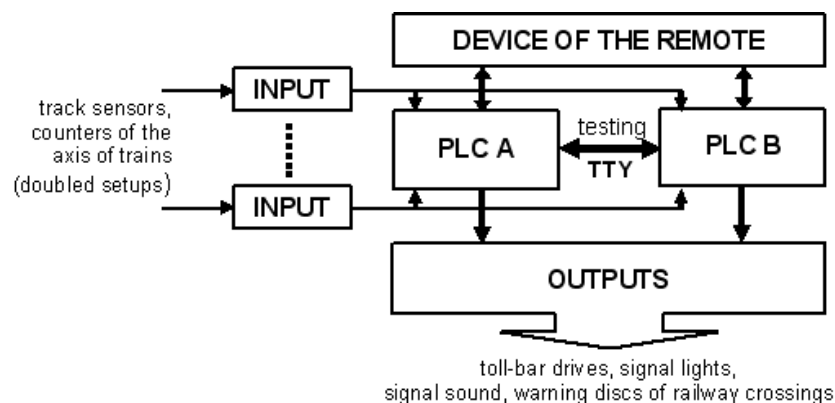
Fig. 1. Example of the configuration of PLC drivers in the automatic SPA-4 system of level crossing Rys. 1. Przykład konfiguracji sterowników PLC w systemie samoczynnej sygnalizacji przejazdowej SPA-4
