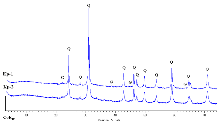
Rys. 1. Dyfratogramy krzemieni z piasków wzgórz morenowych Fig. 1. The X-ray diffractograms of flints form sands in moraine heaps
