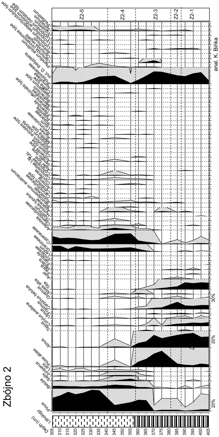
Fig. 3. Pollen diagram – Zbójno 2 core.
