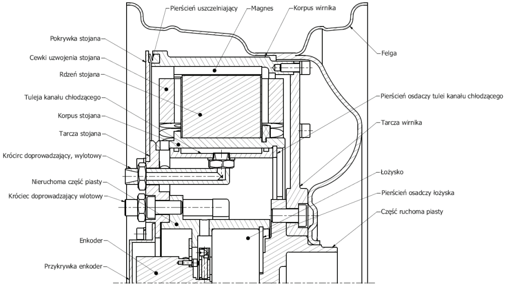
Rys. 1. Przekrój maszyny umieszczonej w kole Fig. 1. Section of the machine placed in the wheel
