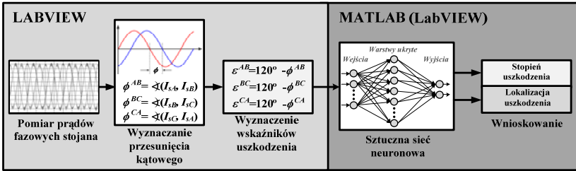
Rys. 4. Neuronowy detektor zwarców zwojowych wykorzystujący metodę analizy przesunięcia kąowego pomiędzy prądami fazowymi stojana Fig. 4. Stator windings fault neural detector based on the phase shift analysis between the stator phase currents
