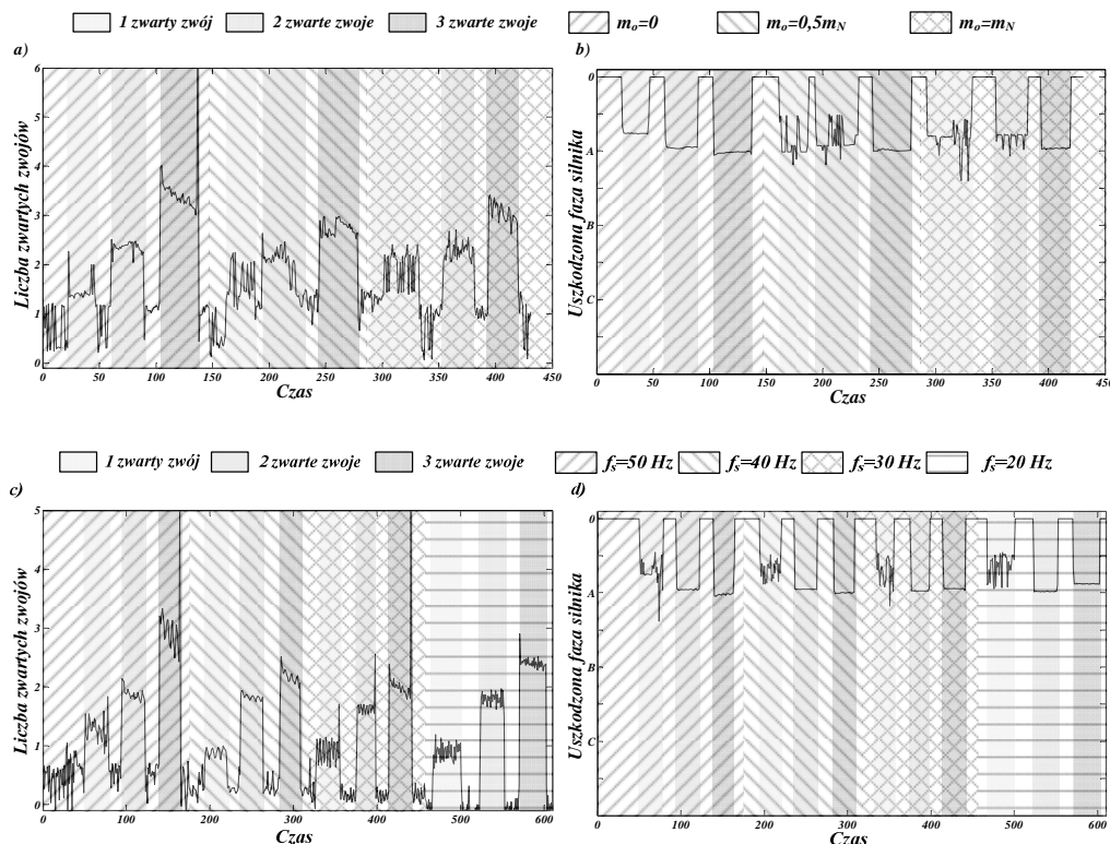
Rys. 5. Odpowiedzi neuronowego detektora uszkodzeń uzwojeń stojana {5-19-2} pracującego on-line przy fizycznym modelowaniu zwarć zwojowych fazy A silnika przy: a) ,b) różnym obciążeniu maszyny dla f_s = 50 Hz i c) ,d) przy różnej wartości częstotliwości napięcia zasilania dla m_o = 0 :
