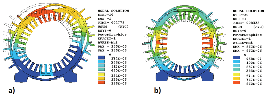
Rys. 7. Postać deformacji U [m] stojana dla modelu A dla wybranych położeń wirnika: a) 10 stopień; b) 30 stopni Fig. 7. Shape of deformation of stator U [m] for model A for selected positions of rotor: a) 10 degree; b) 30 degree
