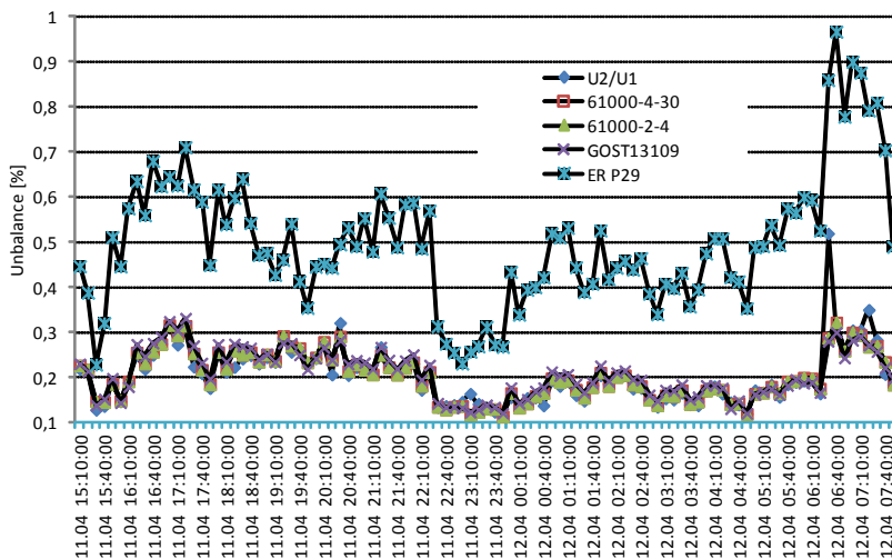
Rys. 8. Współczynnik asymetrii w obliczony z różnych zależności podawanych w normach Fig. 8. Unbalance factor calculated from different formulas given in the standards
