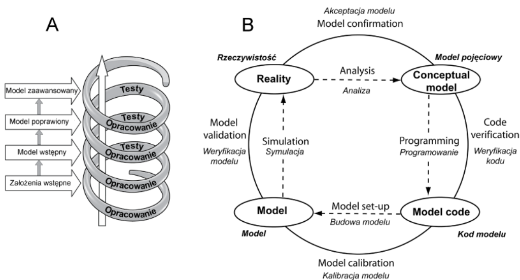
Rys. 1.2. A – Opracowanie modeli UML i schematów XSD dedykowanych określonej dziedzinie jest z konieczności procesem cyklicznym, w którym kolejno postają coraz bardziej dojrzałe wersje. B – Metamodel modeli – podstawowe pojęcia z zakresu modelowania i zachodzące między nimi relacje (Refsgaard, Henriksen, 2004).
