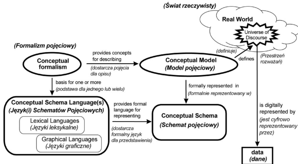
Rys. 1.3. Od rzeczywistości do schematu pojęciowego, opartego na pojęciowym formalizmie i na języku schematów pojęciowych. Cytat z normy ISO 19103 (ISO/TC 211, 2005a) z uzupełnieniami terminów polskich. W tym przypadku jest to tylko model statyczny rzeczywistości.
