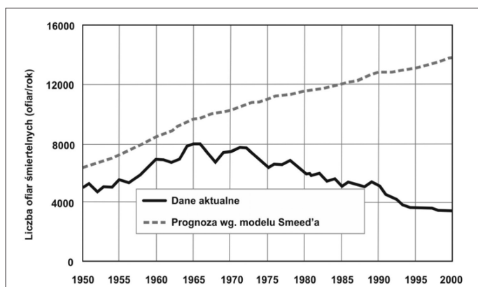
Rys. 1. Prognoza liczby ofiar śmiertelnych w Wielkiej Brytanii według modelu Smeeda
