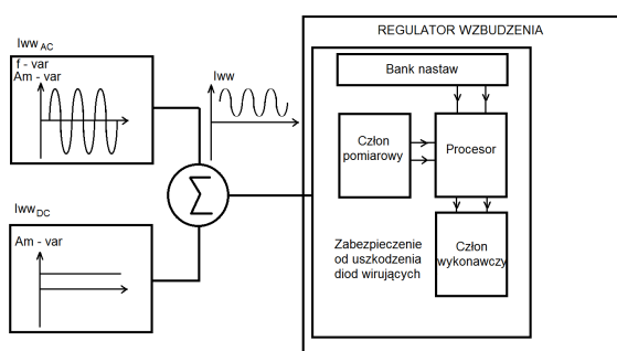
Rys. 5. Schemat blokowy układu do prób wykrywającego uszkodzenia diody we wzbudnicy bezszczotkowej, gdzie: I_{wwAC} , I_{wwDC} – składowe zmienna i stała w prądzie wzbudzenia wzbudnicy I_{ww}
