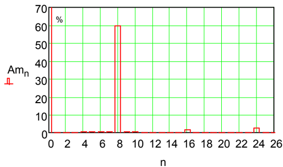
Rys. 4. Wartości harmonicznych w przebiegu jak na rys. 3
