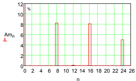
Rys. 2. Wartości harmonicznych w przebiegu jak na rys. 1
