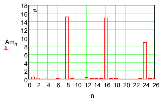
Rys. 7. Wartości harmonicznych w przebiegu jak na rys. 6
