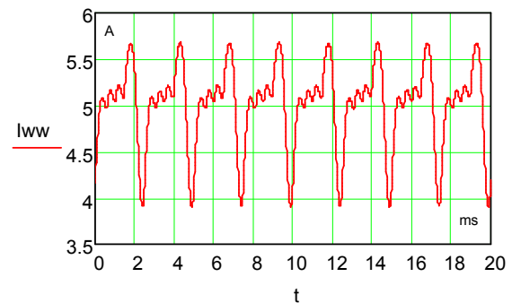
Rys. 1. Przebieg prądu wzbudzenia wzbudnicy z przerwana diodą dla I_{wwsr}=5,0 A
