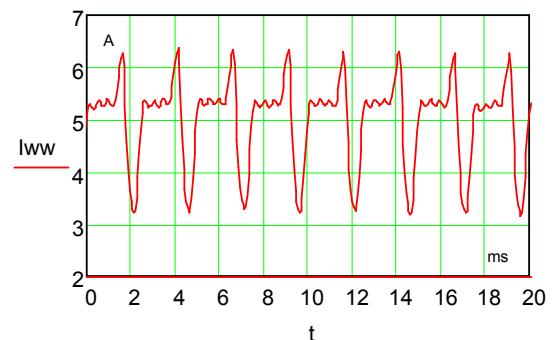
Rys. 6. Przebieg prądu wzbudzenia wzbudnicyz przerwana diodą dla I_{wwsr}=4,995 A
