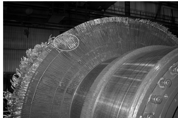
Rys. 4. Widok komutatora. Zaznaczono miejsce zainicjowania zwarcia.
