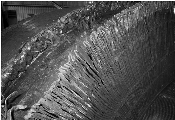
Rys. 2. Uszkodzenie uzwojenia wirnika i chorygiewek komutatora
