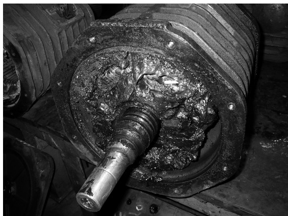
Rys. 6. Nadmierne smarowanie łożyska. Oczyszczona przyczyna źródłowa awarii silnika
