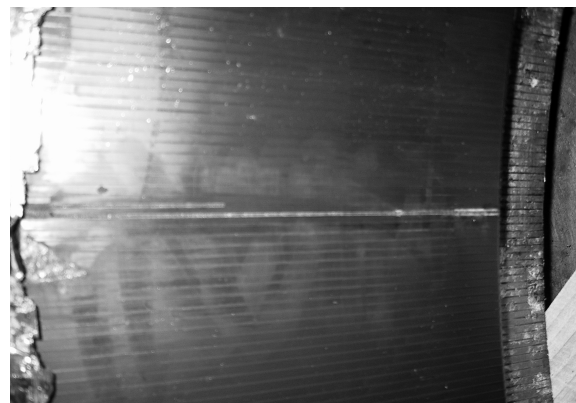
Rys. 5. Widok komutatora po demontażu. Widoczne wyraźnie miejsce zwarcia
