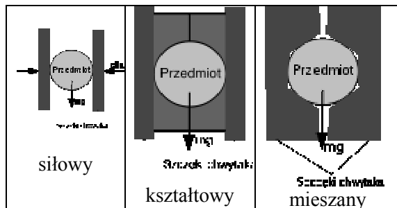
Rys.2. Sposoby trzymania detali przez element wykonawczy [7, 8]
