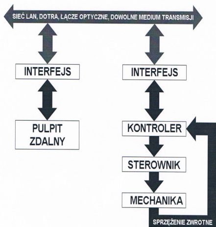
Rys. 6. Schemat blokowy układu sterowania manipulatora [5,6]
