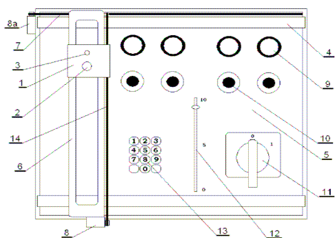
Rys. 4. Widok manipulatora sterującego nałożonego na pulpit sterowniczy [5,6]
