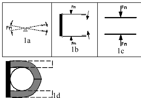
Rys.1. Przykładowe rozwiązania chwytaków manipulatorów: nożycowy - 1a, szczypcowy - 1b oraz imadłowy - 1c. 1d - obejmujący [7]
