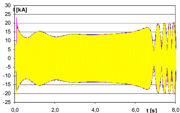
Rys. 5. Prądy stojana podczas zakłócenia
