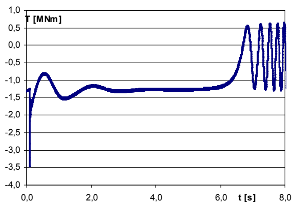
Rys. 6. Moment elektromagnetyczny podczas skokowej zmiany obciążenia
