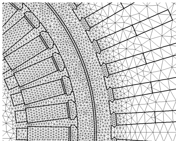
Rys. 2. Fragment siatki dyskretyzacyjnej
