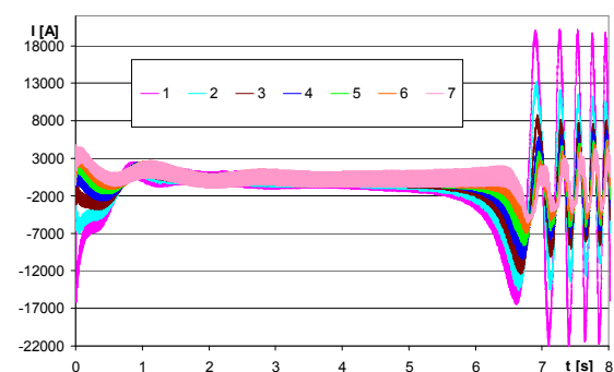
Rys. 7. Prądy w częściach czynnych uzwojenia tłumiającego przy utracie synchronizmu (numeryacja prądów zgodna z rys. 1)
