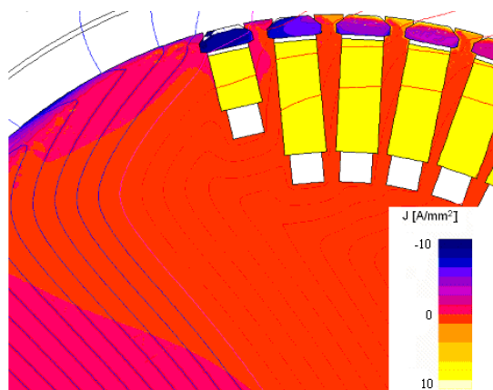
Rys. 9. Rozkład gęstości prądów wirnika przy przejściu w stan pracy niestabilnej
