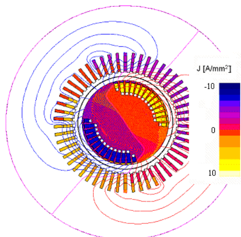
Rys. 8. Rozkład pola magnetycznego oraz gęstości prądów przy przejściu w stan pracy niestabilnej
