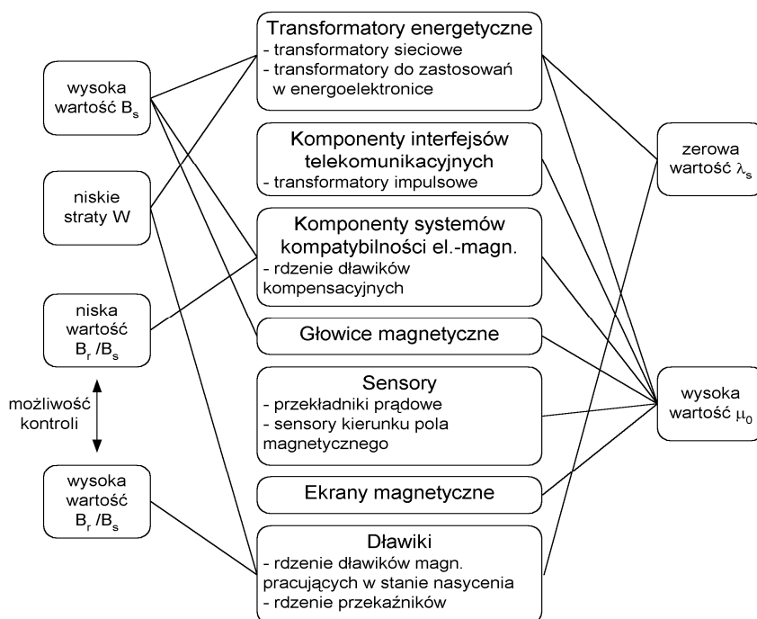
Rys. 3. Właściwości magnetyczne istotne z aplikacyjnego punktu widzenia oraz obszary zastosowań materiałów nanokrystalicznych Źródło: opracowanie własne na podstawie [5]
