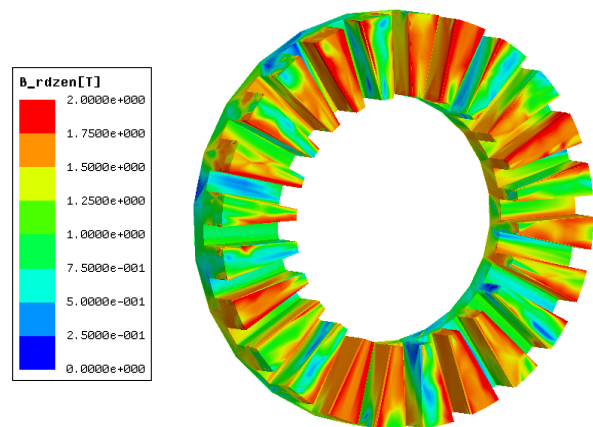
Rys. 14. Rozkład indukcji magnetycznej w zębach w chwili maksymalnego przepływu strumienia pola stojana dla prądu I=115 A.
