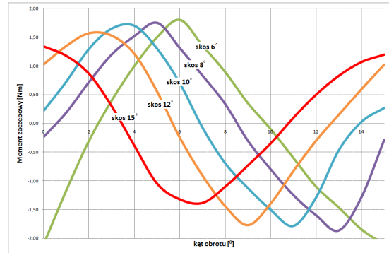
Rys.11. Charakterystyka momentu zaczepowego w funkcji kąta obrotu wirnika dla różnych skosów magnesu i emb=0.7
