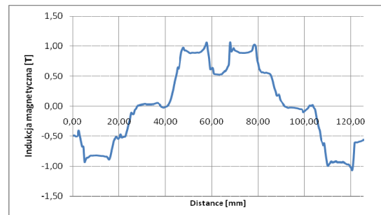
Rys.7. Rozkład indukcji magnetycznej od magnesów trwałych w szczeliny powietrznej na promieniu średnim
