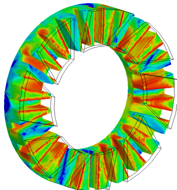
Rys.10. Rozkład indukcji magnetycznej w zębach stojana z widocznymi konturami magnesów trwałych
