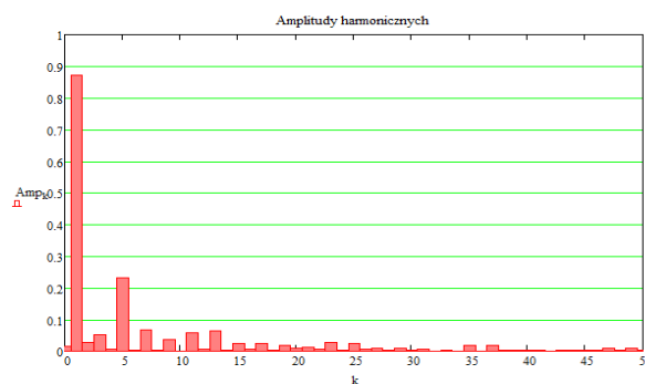
Rys.8. Amplitudy poszczególnych harmonicznych indukcji magnetycznej w szczeliny powietrznej na promieniu średnim
