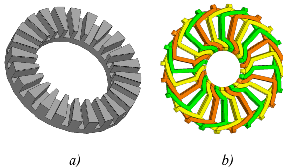
Rys.2. a) Model rdzenia stojana b) model uzwojenia stojana
