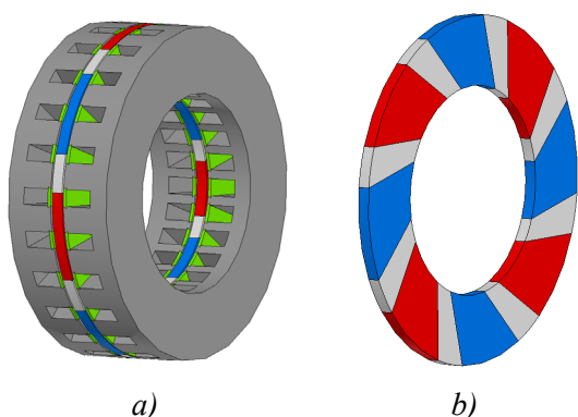
Rys.1. a) Model obwodu magnetycznego silnika tarczowego z wirnikiem wewnętrznym b) model wirnika
