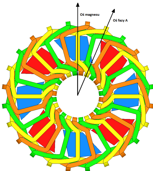
Rys. 13. Ustawienie położenia wirnika względem uzwojenia stojana dla zadanych wymuszeń prądowych
