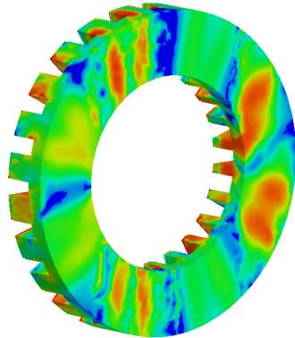
Rys.9. Rozkład indukcji magnetycznej w jarzmie stojana
