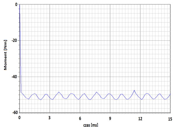
Rys. 15. Przebieg momentu elektromagnetycznego dla prądu fazowego I=115 A.
