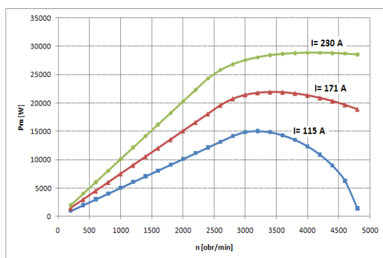
Rys.5. Moc mechaniczna silnika w funkcji prędkości obrotowej dla różnych wartości prądów fazowych
