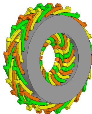
Rys.3. Model zaprojektowanego obwodu elektromagnetycznego silnika tarczowego
