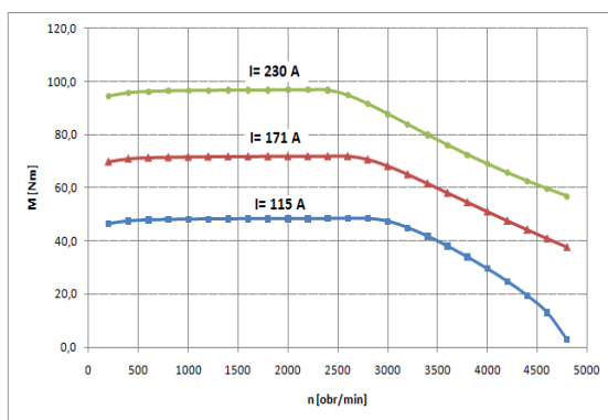
Rys.4. Moment na wale silnika w funkcji prędkości obrotowej dla różnych wartości prądów fazowych
