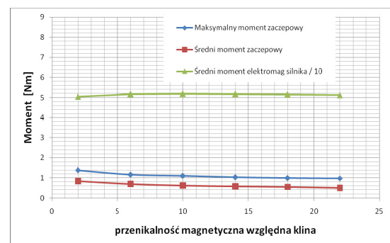
Rys.12. Charakterystyki momentów w funkcji przenikalności magnetycznej klina dla omawianego modelu silnika.
