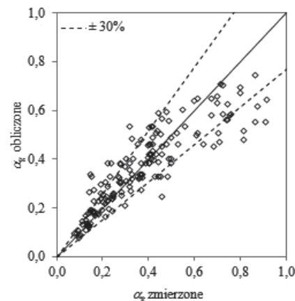
Rys. 3. Porównanie udziału objętościowego obliczonego ze zmierzonym dla przepływu dwufazowego gaz – ciecz we wszystkich badanych minikanalach
