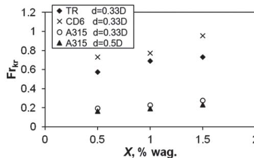
Rys. 1. Zależność Fr_{kr} = f(X) dla układu woda destylowana – cząstki ciała stałego o średniej średnicy d_z = 212 \mu\text{m} i mieszadła: turbinowego Rushtona (TR), turbinowego Smitha (CD 6) oraz A315, gdzie d = 0,33D lub d = 0,5D
