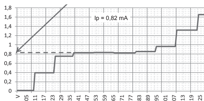
Rys. 1. Przykład rejestracji prądu plateau
