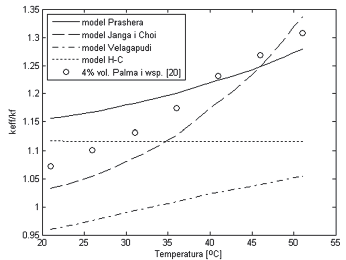
Rys. 6. Porównanie przewidywań badanych modeli z danymi eksperymentalnymi [20] dla 4% stężenia objętościowego Al_2O_3 w wodzie
