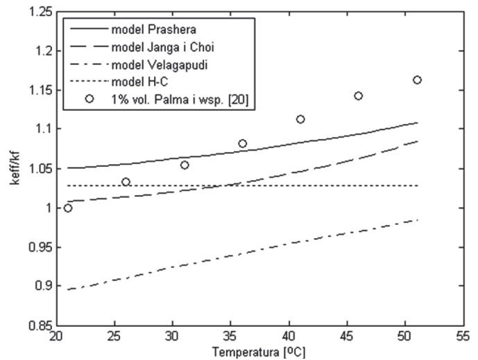
Rys. 5. Porównanie przewidywań badanych modeli z danymi eksperymentalnymi [20] dla 1% stężenia objętościowego Al_2O_3 w wodzie
