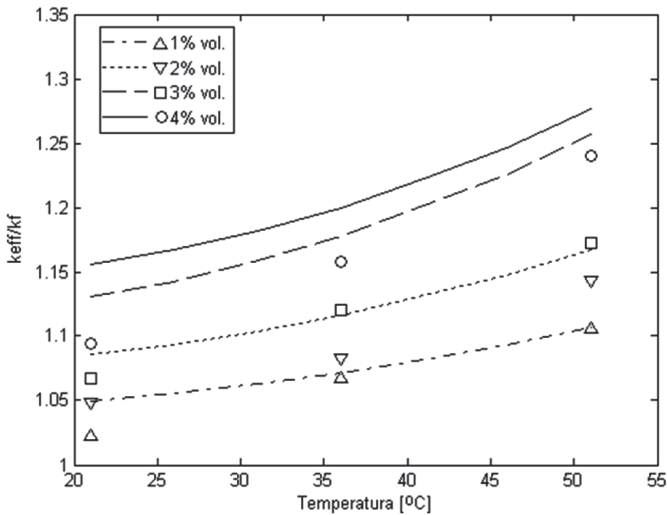
Rys. 2. Przewidywania modelu Prashera (linie) w porównaniu z danymi eksperymentalnymi (punkty) Dasa i wsp. [13] dla czterech różnych stężeń objętościowych cząstek Al_2O_3 w wodzie
