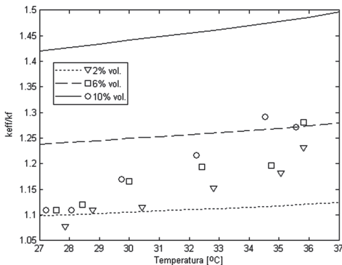
Rys. 4. Przewidywania Prashera (linie) w porównaniu z danymi eksperymentalnymi (punkty) Li i Petersona [21] dla trzech różnych stężeń objętościowych cząstek Al_2O_3 w wodzie
