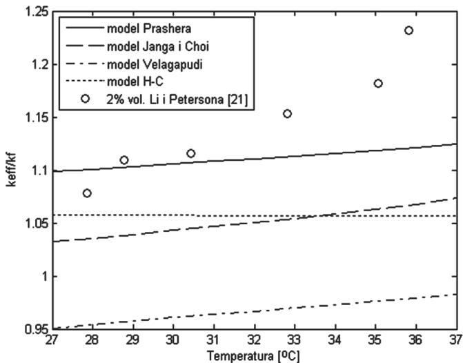
Rys. 7. Porównanie przewidywań badanych modeli z danymi eksperymentalnymi [21] dla 2% stężenia objętościowego \text{Al}_2\text{O}_3 w wodzie
