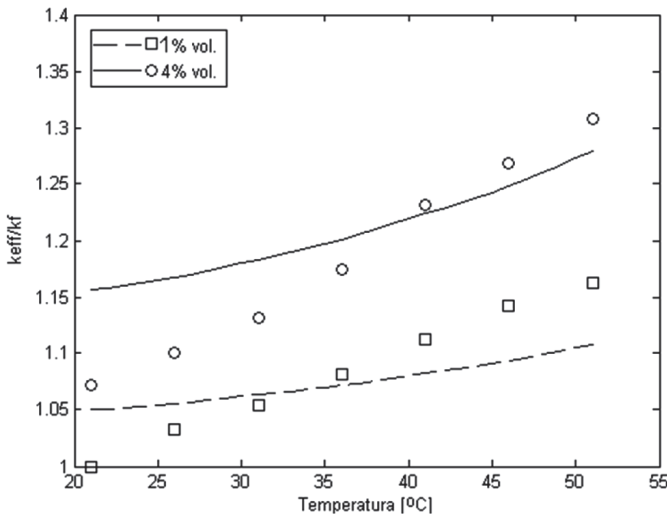
Rys. 3. Przewidywania Prashera (linie) w porównaniu z danymi eksperymentalnymi (punkty) Palma i wsp. [20] dla dwóch różnych stężeń objętościowych cząstek Al_2O_3 w wodzie
