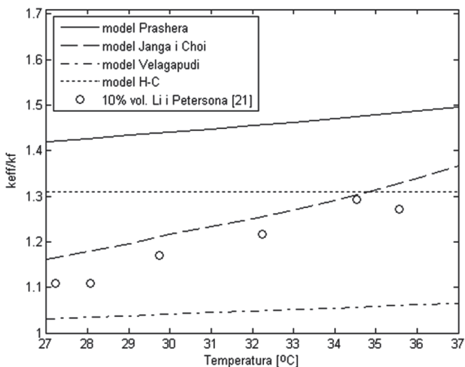
Rys. 9. Porównanie przewidywań badanych modeli z danymi eksperymentalnymi [21] dla 10% stężenia objętościowego \text{Al}_2\text{O}_3 w wodzie
