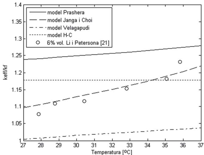
Rys. 8. Porównanie przewidywań badanych modeli z danymi eksperymentalnymi [21] dla 6% stężenia objętościowego \text{Al}_2\text{O}_3 w wodzie
