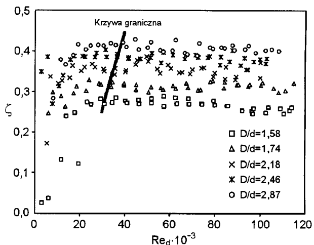
Rys. 3. Zbiorne zestawienie zależności współczynnika strat miejscowych ( \zeta ) od liczby Reynoldsa ( Re_d )
