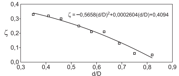
Rys. 5. Zależność współczynnika strat miejscowych ( \zeta ) od stopnia zwężenia rury ( d/D ) Fig. 5. Resistance coefficient ( \zeta ) related to pipe contraction ( d/D )
