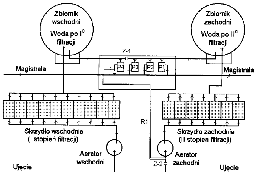
Rys. 1. Schemat stacji uzdatniania wód podziemnych „Letniki” po modernizacji (przed modernizacją nie było rurociągu R1 oraz zasuw Z-1, a zasawa Z-2 była otwarta)
