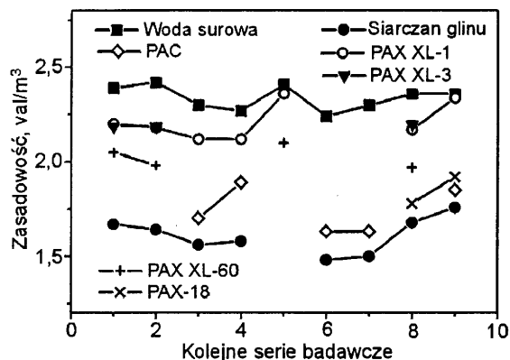
Rys. 4. Długookresowe wartości zasadowości wody surowej i po koagulacji badanymi koagulantami w dawce podstawowej 80 \text{ g/m}^3
