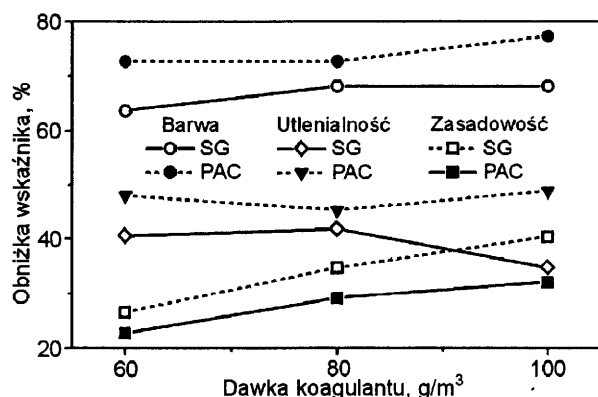
Rys. 1. Porównanie skuteczności siarczanu glinu (SG) i preparatu PAC w obniżaniu barwy, utleniałości i zasadowości
