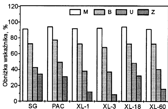
Rys. 2. Porównanie obniżania mętności (M), barwy (B), utlenialności (U) i zasadowości ogólnej (Z) wody w procesie koagulacji dla wszystkich testowanych koagulantów w dawce podstawowej 90 \text{ g/m}^3
