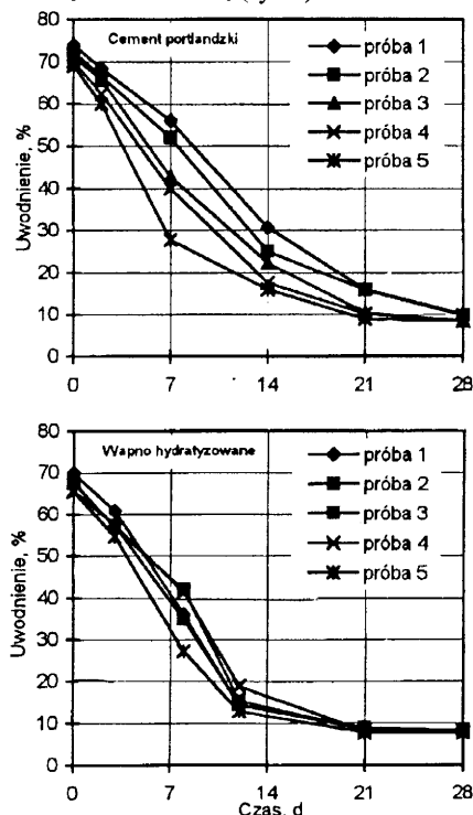
Rys. 1. Przebieg zmian uwodnienia osadów ściekowych podczas ich zestalania cementem i wapnem (pr. 1 – 10% sm osadu, pr. 2 – 20% sm osadu, pr. 3 – 30% sm osadu, pr. 4 – 40% sm osadu, pr. 5 – 50% sm osadu)
