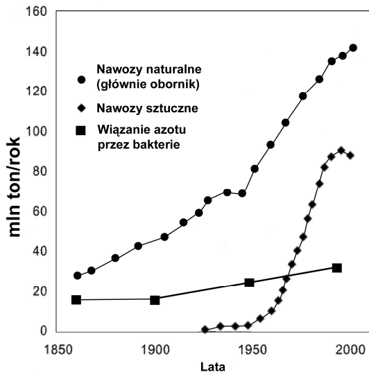
Rys. 10. Charakterystyka przepływu do geokoosystemu Ziemi związków azotowych podawanych w postaci nawozów w latach 1850 – 2000.
