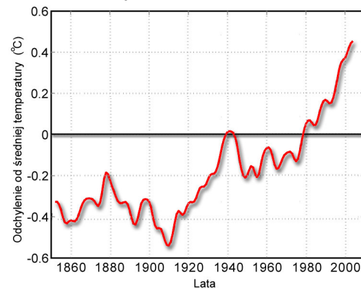
Rys.3. Charakterystyka odchylenia średniej temperatury powierzchni Ziemi w poszczególnych latach od średniej za lata 1960-90.
