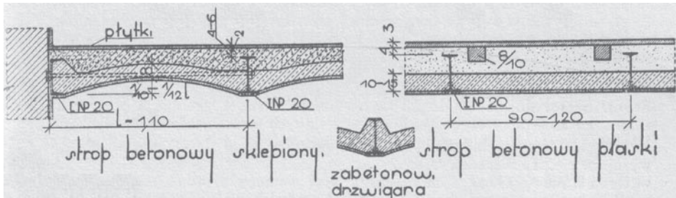
Rys. 18. Strop betonowy odcinkowy, strop płaski niezbrojony.
