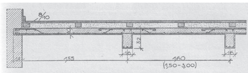
Rys. 21. Strop żebrzowy.
