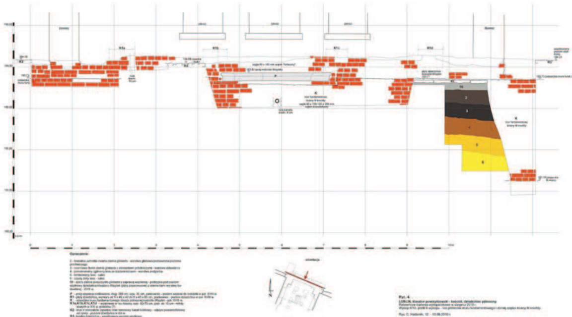
Ryc. 4. Lublin, klasztor powizytkowski, kościół. Ratownicze badania wykopaliskowe w sierpniu 2010 r. Wykop 6/10, profil S wykopu – lico północne muru fundamentowego i dolnej części ściany N kruchty. Rys. C. Hadamik, 12-13.08.2010 r. Fig. 4. Lublin, post-Visitationist monastery, church. Rescue excavations in August 2010. Dig 6/10, profile S of the dig – north face of the foundation wall and the lower section of the N wall of the porch. Drawn by C. Hadamik, 12-13.08.2010
