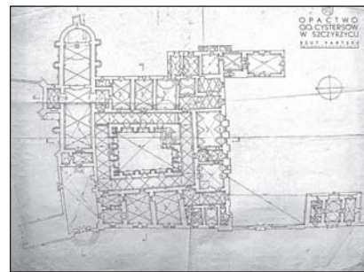
Ryc. 7. Plan parteru zabudowań klasztornych, inwentaryzacja wykonana przez Bohdana Lisowskiego w ramach prac Katedry i Zakładu Historii Architektury Polskiej Politechniki Krakowskiej w roku 1944. Inwentaryzacja w zbiorach archiwum Instytutu Historii Architektury i Konserwacji Zabytków Politechniki Krakowskiej
