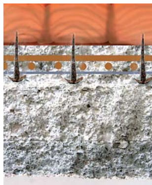
Ryc. 4. Uniwersytet Wrocławski, Aula Leopoldina; schemat układu warstw w strefie sklepienia Fig. 4. University of Wrocław, Aula Leopoldina; scheme of layer arrangement in the vault zone
