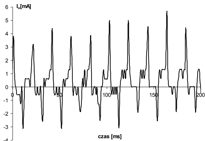
Rys. 7. Przebieg prądu upływowego w ograniczniku zmierzony przy napięciu U=345 \text{ V} > U_c=275 \text{ V}
