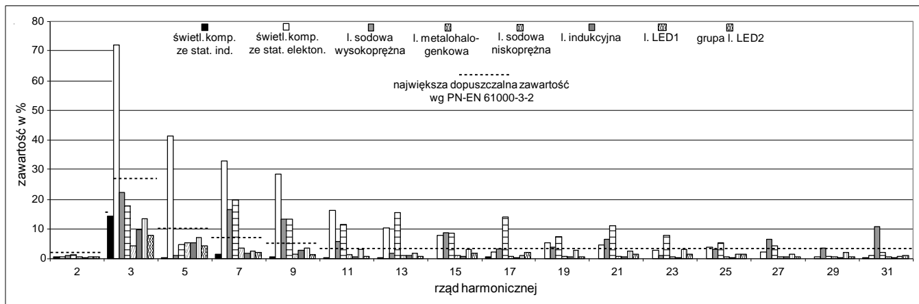
Rys. 9. Udział 2. harmonicznej i harmoniczných nieparzystych od 3. do 31. w analizowanych przebiegach prądu obciążenia oraz największe wartości wyższych harmoniczných dopuszczone przez normę [15]
