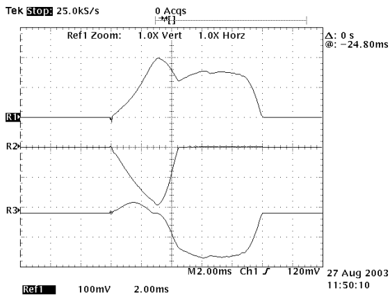
Rys. 4. Oscylogram jednofazowego wyłączenia trójfazowego zwarcia łukowego przy pomocy bezpiecznika WT 160; napięcie probiercze U_b=460 V, spodziewany prąd zwarciov I_k=11,7 kA, kąt fazowy napięcia \psi=27^\circ , d=50 mm, Cu.; R1 – prąd i_{L1} , R2 – prąd i_{L2} , R3 – prąd i_{L3} , stała k_f=4 kA/dz.
