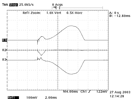
Rys. 5. Oscylogram jednofazowego wyłączenia trójfazowego zwarcia łukowego przy pomocy wyłącznika WACH; U_b=403 V, spodziewany prąd zwarciov I_k=11,7 kA, prąd dyskryminatora 1000 A, d=60 mm, Al; R1 – prąd i_{L1} , R2 – prąd i_{L2} , R3 – prąd i_{L3} , stała k_f=4 kA/dz.
