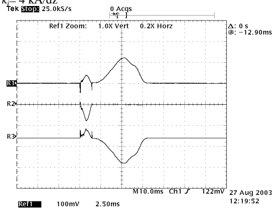
Rys. 6. Oscylogram jednofazowego wyłączenia trójfazowego zwarcia łukowego przy pomocy wyłącznika WACH; napięcie probiercze U_b=403 V, spodziewany prąd zwarciov I_k=19,7 kA, prąd dyskryminatora 1100 A, d=60 mm, Al; R1 – prąd i_{L1} , R2 – prąd i_{L2} , R3 – prąd i_{L3} , stała k_f=4 kA/dz.
