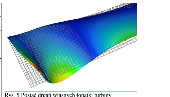
Rys. 5 Postać drgań własnych łopatki turbiny
