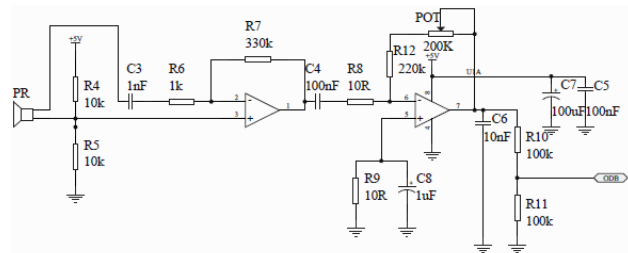
Rys. 2. Schemat ideowy układu odbiornika ultradźwiękowego
