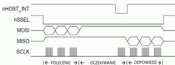
Rys. 5. Procedura komunikacji między modułem ZigBee i hostem
