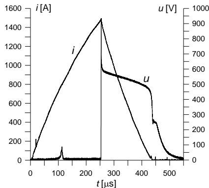
Rys. 2. Przebieg prądu i napięcia CHCL
