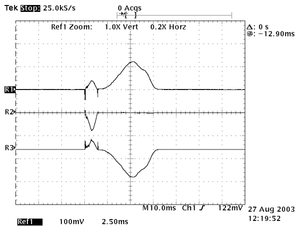
Rys. 6. Oscylogram jednofazowego wyłączenia trójfazowego zwarcia łukowego przy pomocy wyłącznika WACH; napięcie probiercze U_b=403 V, spodziewany prąd zwarcioowy I_k=19,7 kA, prąd dyskryminatora 1100 A, d=60 mm, Al; R1 – prąd i_{L1} , R2 – prąd i_{L2} , R3 – prąd i_{L3} , stała k_i= 4 kA/dz.
