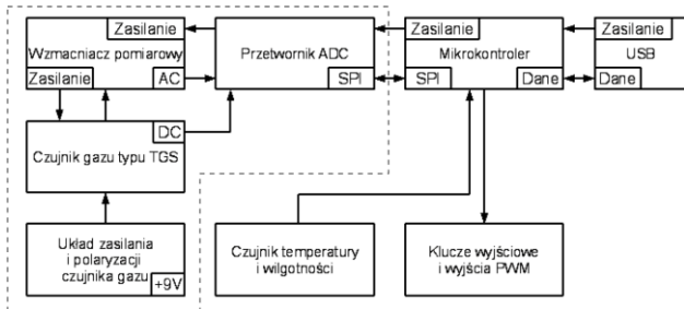
Rys. 2. Schemat blokowy urządzenia
