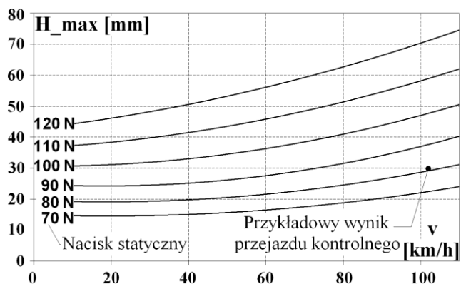
Rys. 17. Charakterystyki uniesienia przewodu jezdnej w zależności od siły statycznej odbieraka i prędkości pojazdu
