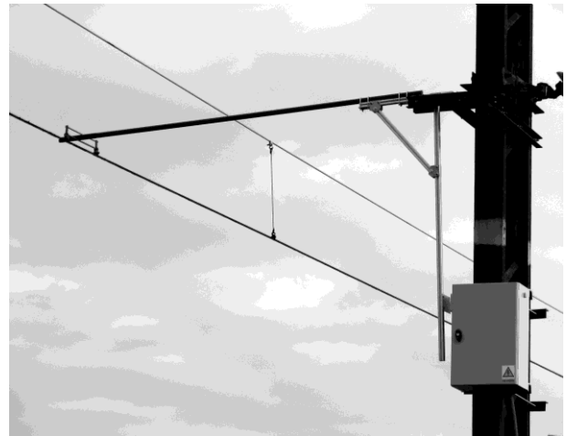
Rys. 8. Układu pomiaru uniesienia przewodu jezdnego
