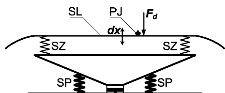
Rys. 11. Dynamiczna współpraca sieci z odbierakiem prądu, gdzie: F_d – dynamiczna siła stykowa, dx – przemieszczenie ślizgacza, SL – łożysko, PJ – przewód trakcyjnej, SZ – sprężyna zawieszenia ślizgacza, SP – sprężyny unoszące odbierak
