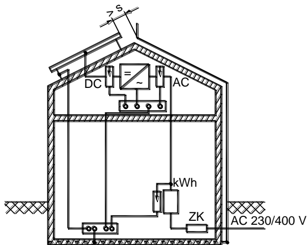
Rys. 5. Ochrona przeciwprzebieciowa systemów PV na dachu budynku z instalacją odgromową z zachowaniem bezpiecznego odstępu izolacyjnego s , =/~ – falownik, ZK – złącze kablowe
