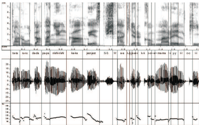
Fig. 7. Spectrogram of the synthesized utterance: 'Ta ruda panienska jest szwagierka Marylki'
