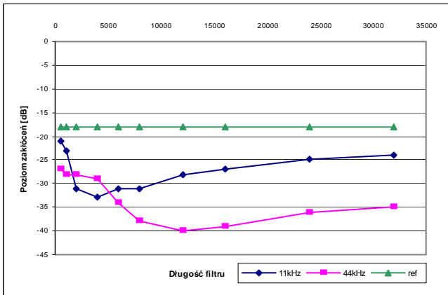
Rys. 4. Wpływ zmiennej długości stosowanego filtra adaptacyjnego na stopień tłumienia zakłóceń dla dwóch częstotliwości próbkowania sygnału. Kolorem zielonym oznaczony poziom zakłócenia w nagraniu.
