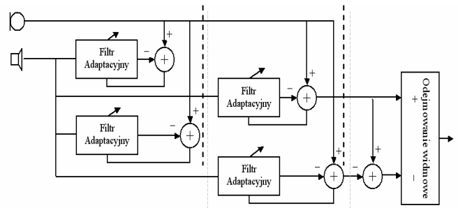
Rys. 6. Schemat blokowy opracowanego algorytmu. Można wyróżnić trzy główne części: filtracja wstępna, filtracja właściwa, odejmowanie widmowe
